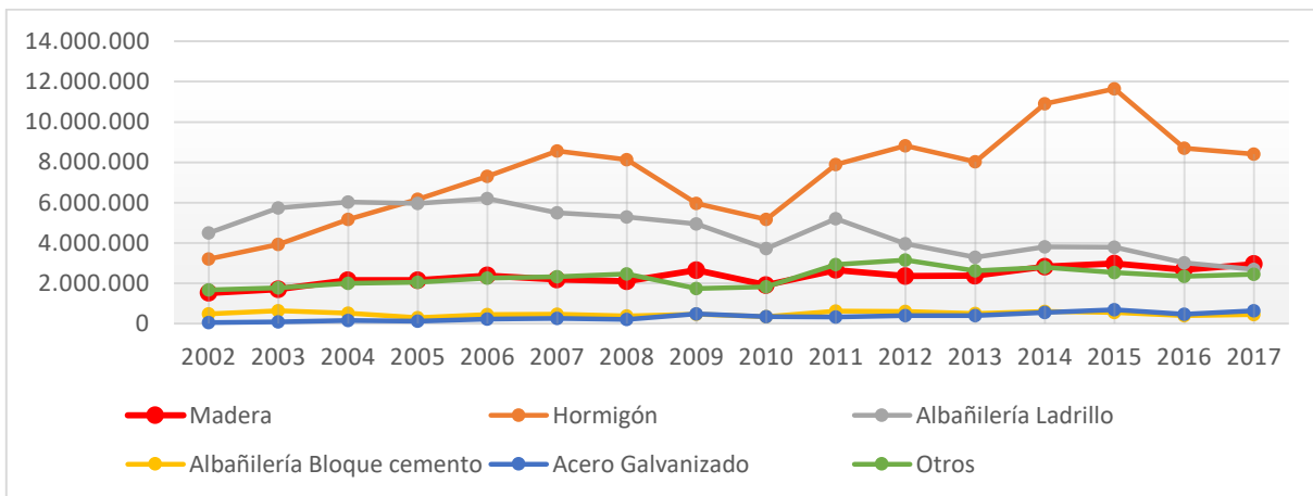
Gráfico 17: Superficie autorizada (m2) cada año según materialidad predominante
