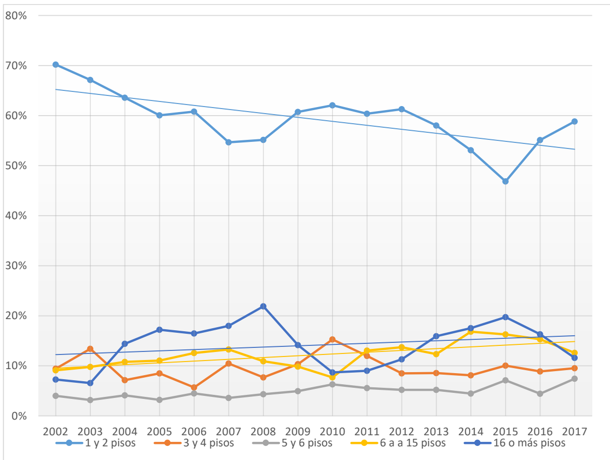
Gráfico 26: Distribución de superficie autorizada expresada en porcentaje según número de pisos para la Zona Centro
