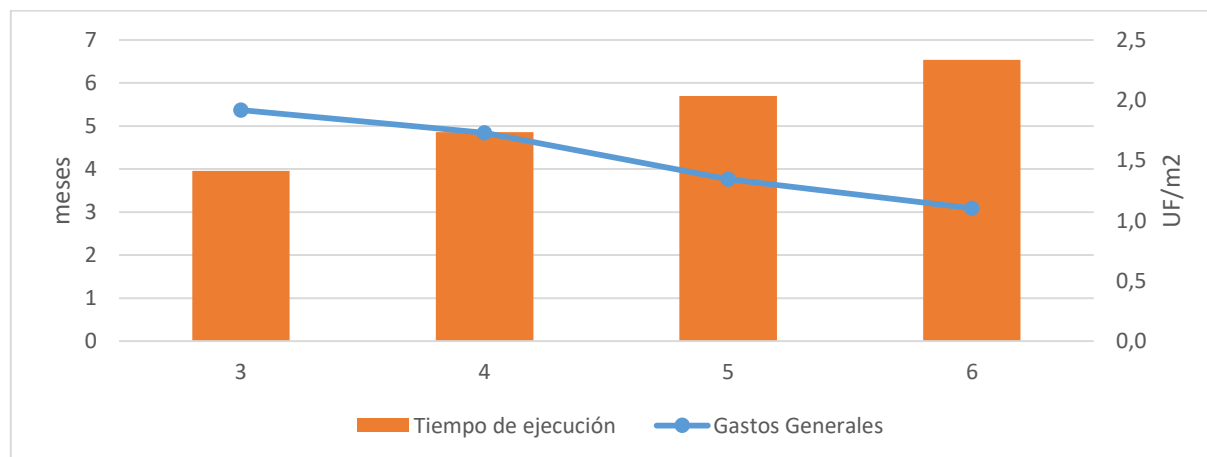
Gráfico 33: Tiempos de ejecución y costos de Gastos Generales (UF/m 2 )
