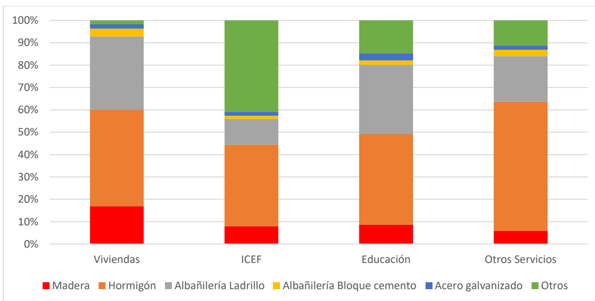
Gráfico 5: Porcentaje de participación de cada materialidad para los 4 destinos.
