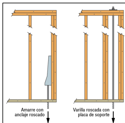
Figura 6: Amarre con anclaje roscado (HD) y anclaje con varilla roscada (ATS)
