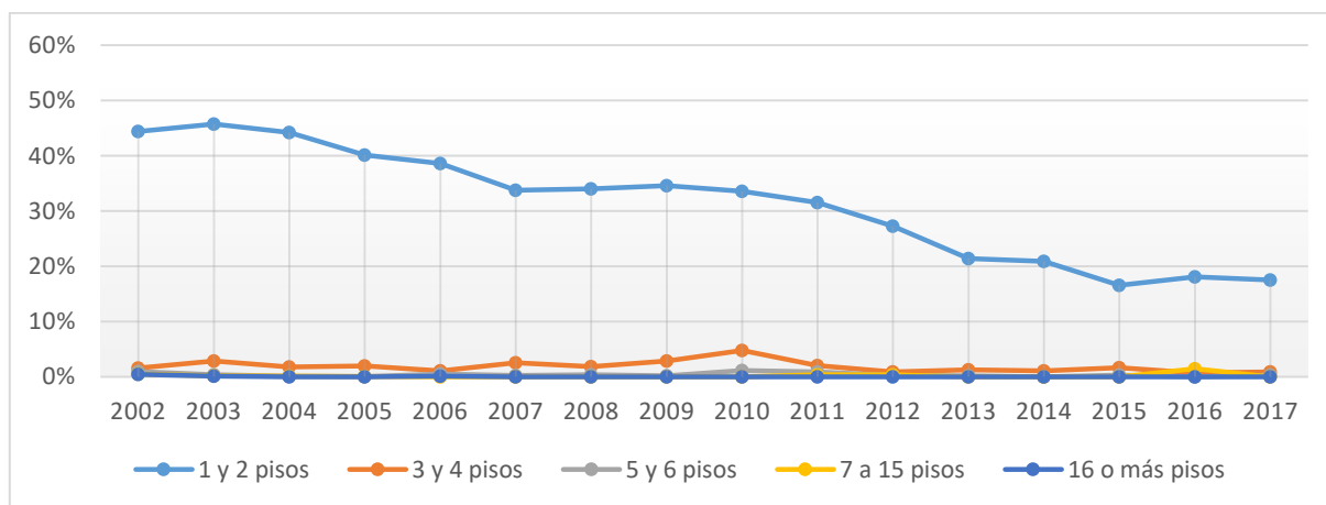
Gráfico 12: Superficie autorizada (m2) expresada en porcentaje para cada año, según agrupación en n° de pisos en destino Vivienda para materialidad predominante Albañilería ladrillo
