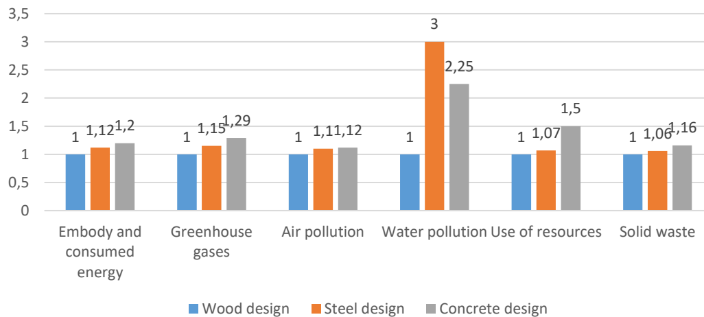
Gráfico 1: Efectos contenidos relativo de la construcción en madera (normalizado a que el valor de la madera es 1).
