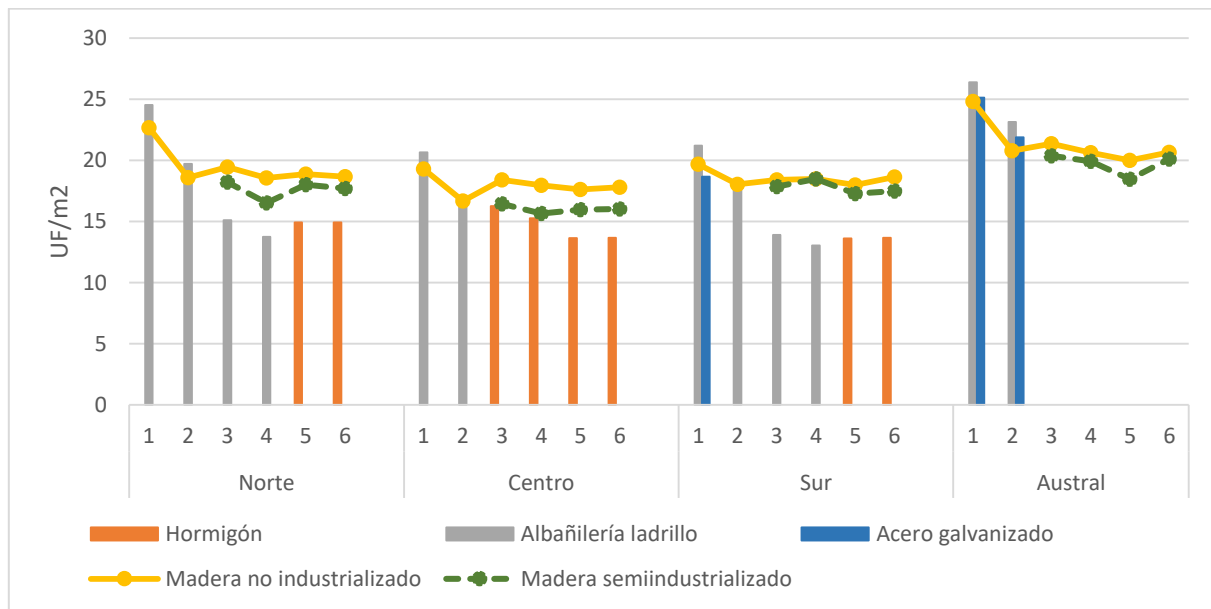
Gráfico 34: Costos Netos (UF/m2) distintas materialidades no industrializado y semiindustrializado
