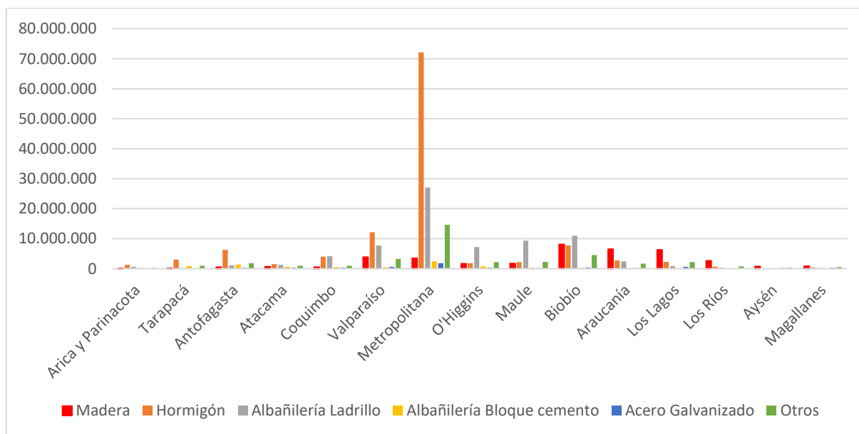
Gráfico 19: Superficie autorizada (m2) para cada región según materialidad predominante
