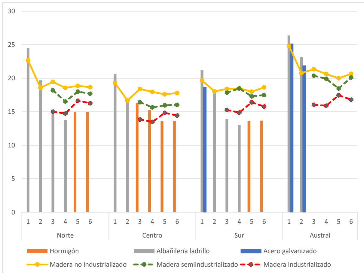
Gráfico 35: Costos Netos (UF/m 2 ) en distintas materialidades y grados de industrialización
