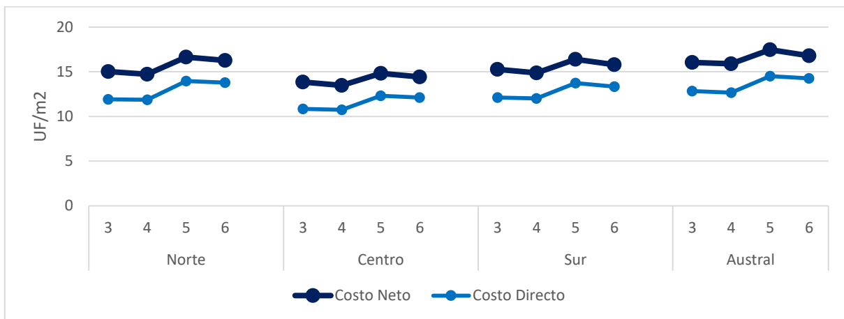
Gráfico 30: Costos Netos y costos directos (UF/m 2 ) según materialidad, cantidad de pisos y Zonificación
