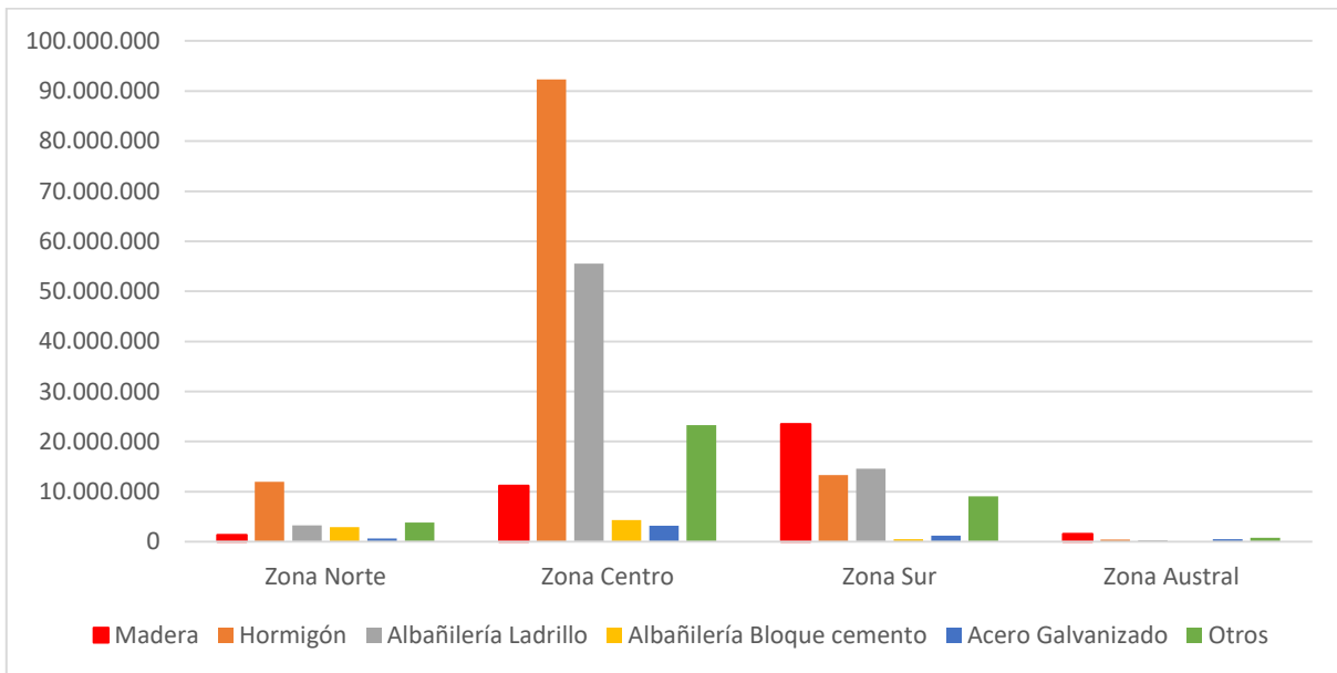
Gráfico 24: Superficie autorizada (m2) para cada Zona según materialidad predominante
