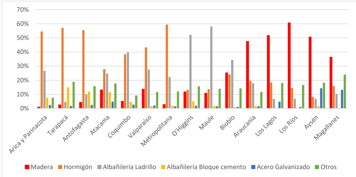
Gráfico 20: Superficie autorizada expresada en porcentaje para cada región según materialidad predominante
