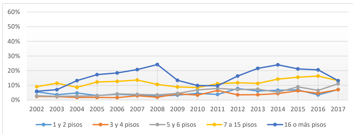
Gráfico 11: Superficie autorizada (m2) expresada en porcentaje para cada año, según agrupación en n° de pisos en destino Vivienda para materialidad predominante Hormigón
