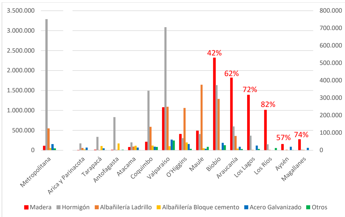
Gráfico 21: Superficie autorizada para destino Vivienda (m2) para cada región según materialidad predominante año 2017
