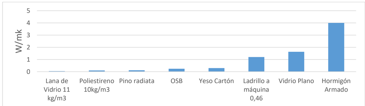
Gráfico 2: Comparación de Conductividades Térmicas en distintas materialidades
