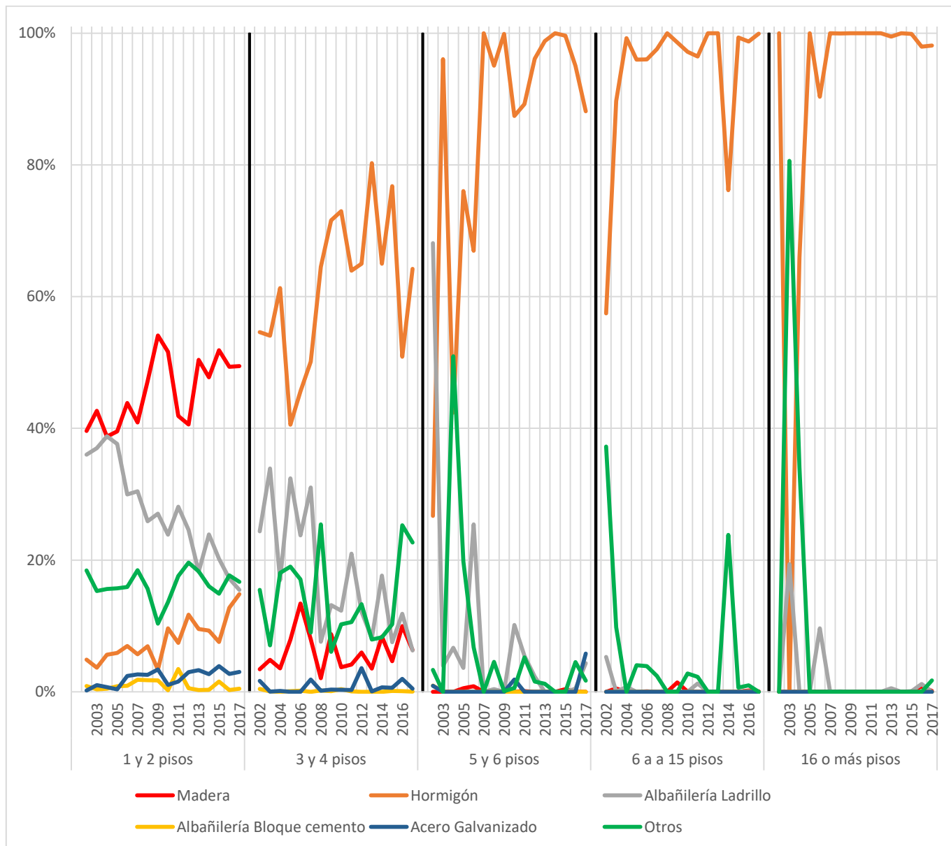
Gráfico 29: Distribución de superficie autorizada según materialidad y número de pisos en la Zona Sur
