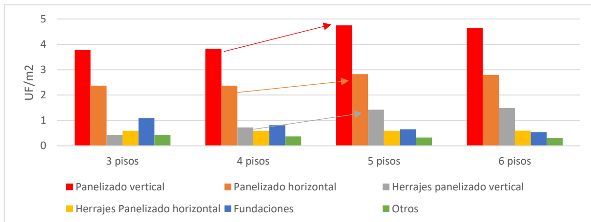
Gráfico 32: Costos detallados de Obra gruesa (UF/m 2 ) (promedio de las cuatro zonas)
