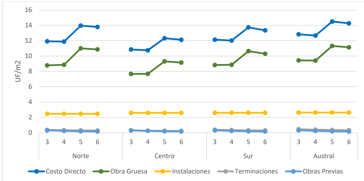
Gráfico 31: Costos Obras Previas, Obra Gruesa, Terminaciones e Instalaciones (UF/m 2 ) según materialidad, cantidad de pisos y Zonificación
