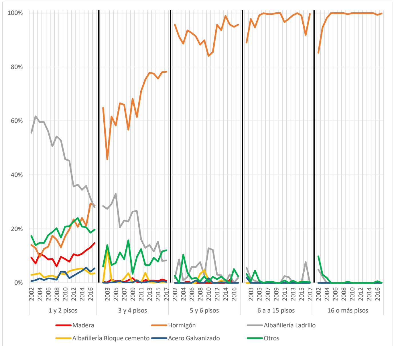
Gráfico 27: Distribución de superficie autorizada según materialidad y número de pisos en la Zona Centro
