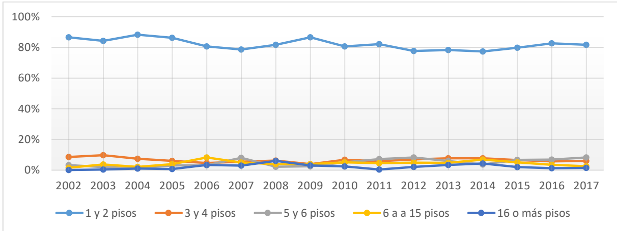
Gráfico 28: Distribución de superficie autorizada expresada en porcentaje según número de pisos para la Zona Sur
